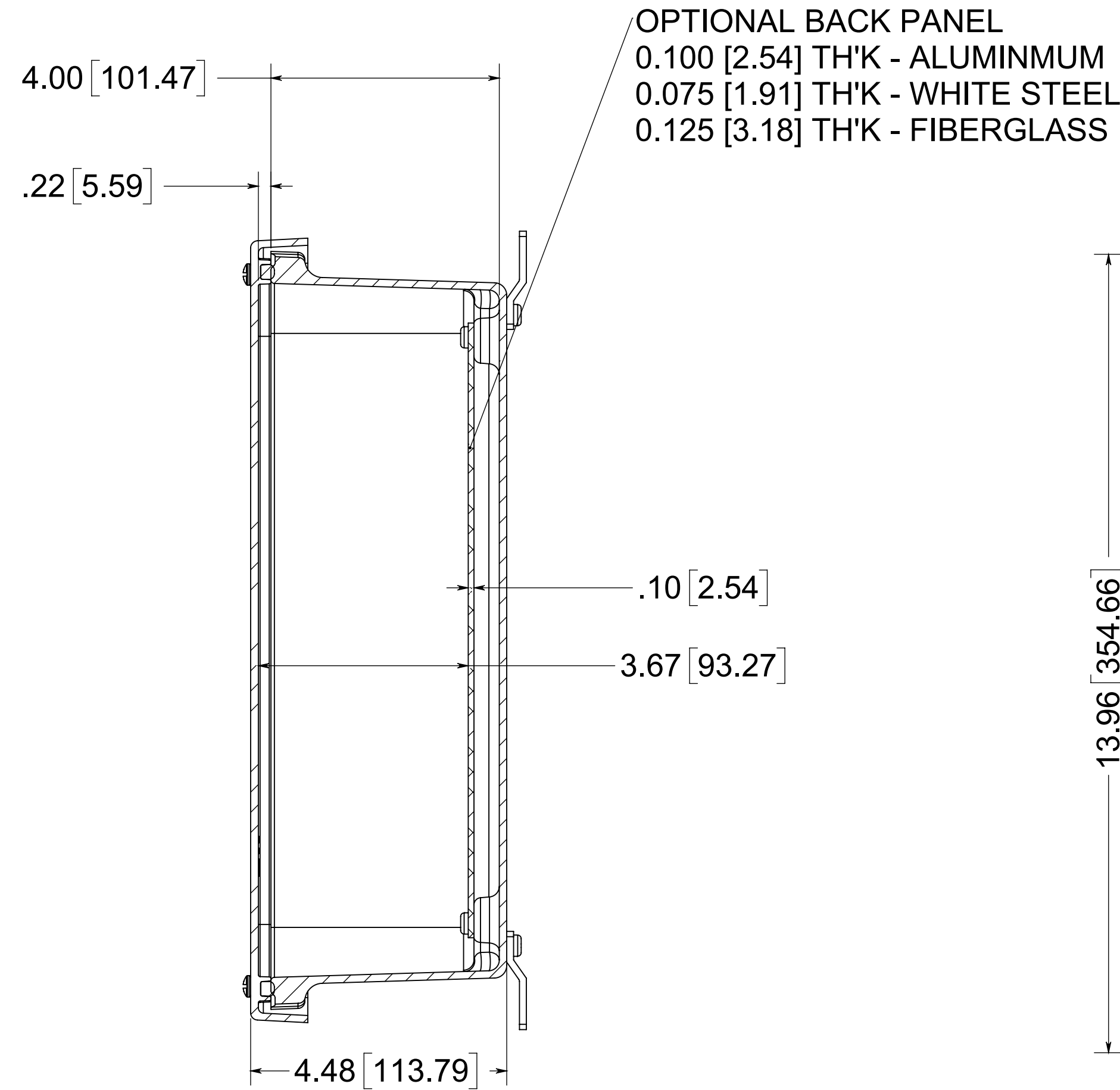
SECTION A-A
