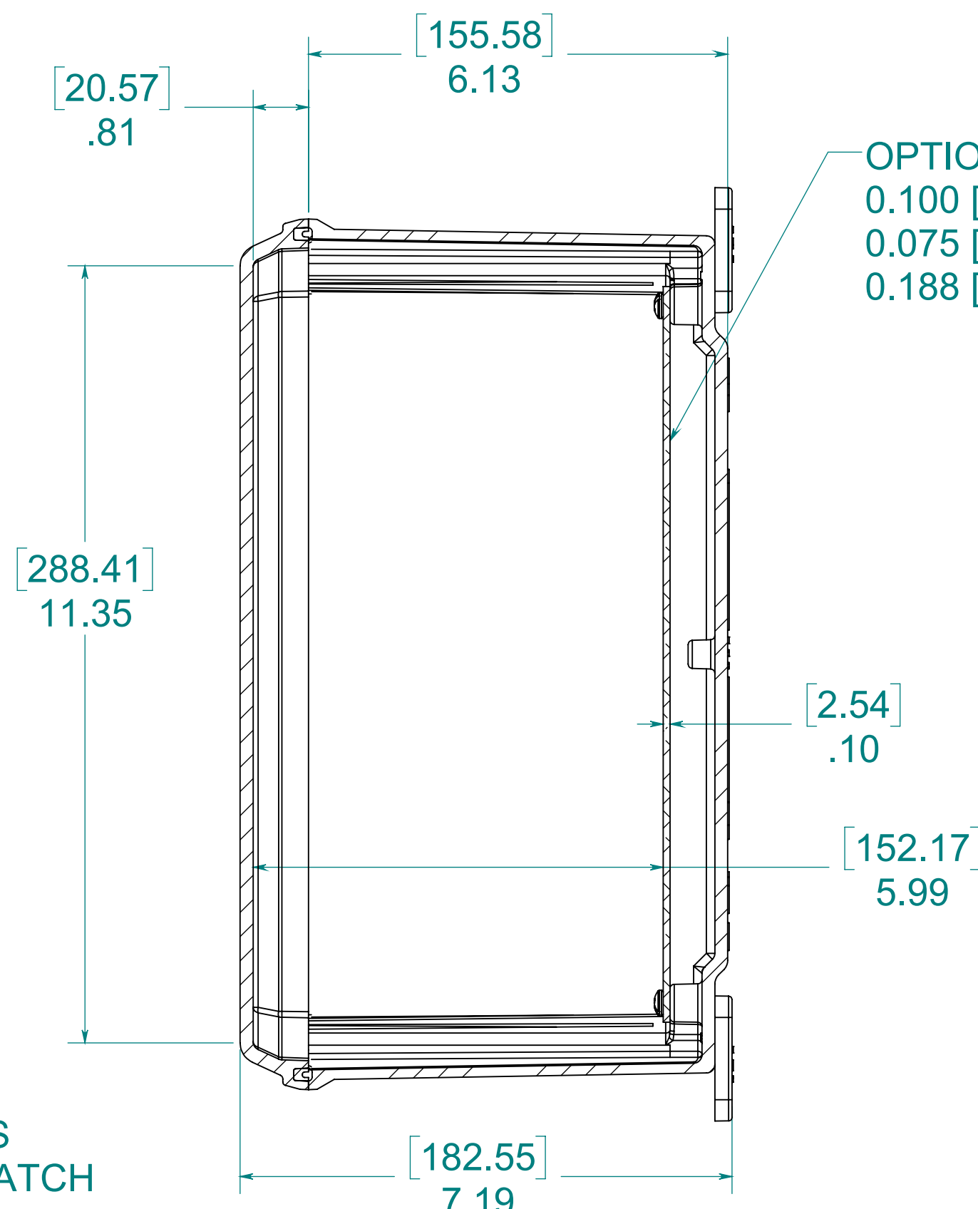
SECTION A-A
