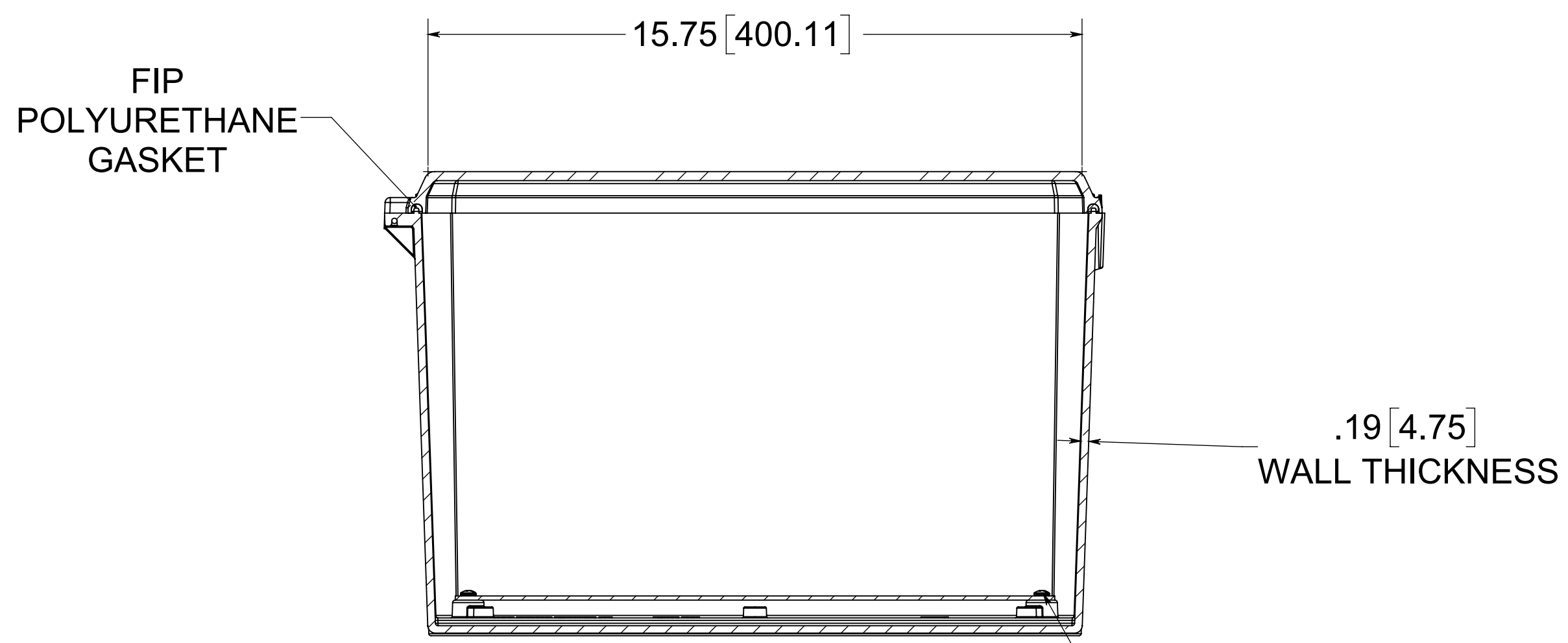
SECTION D-D
