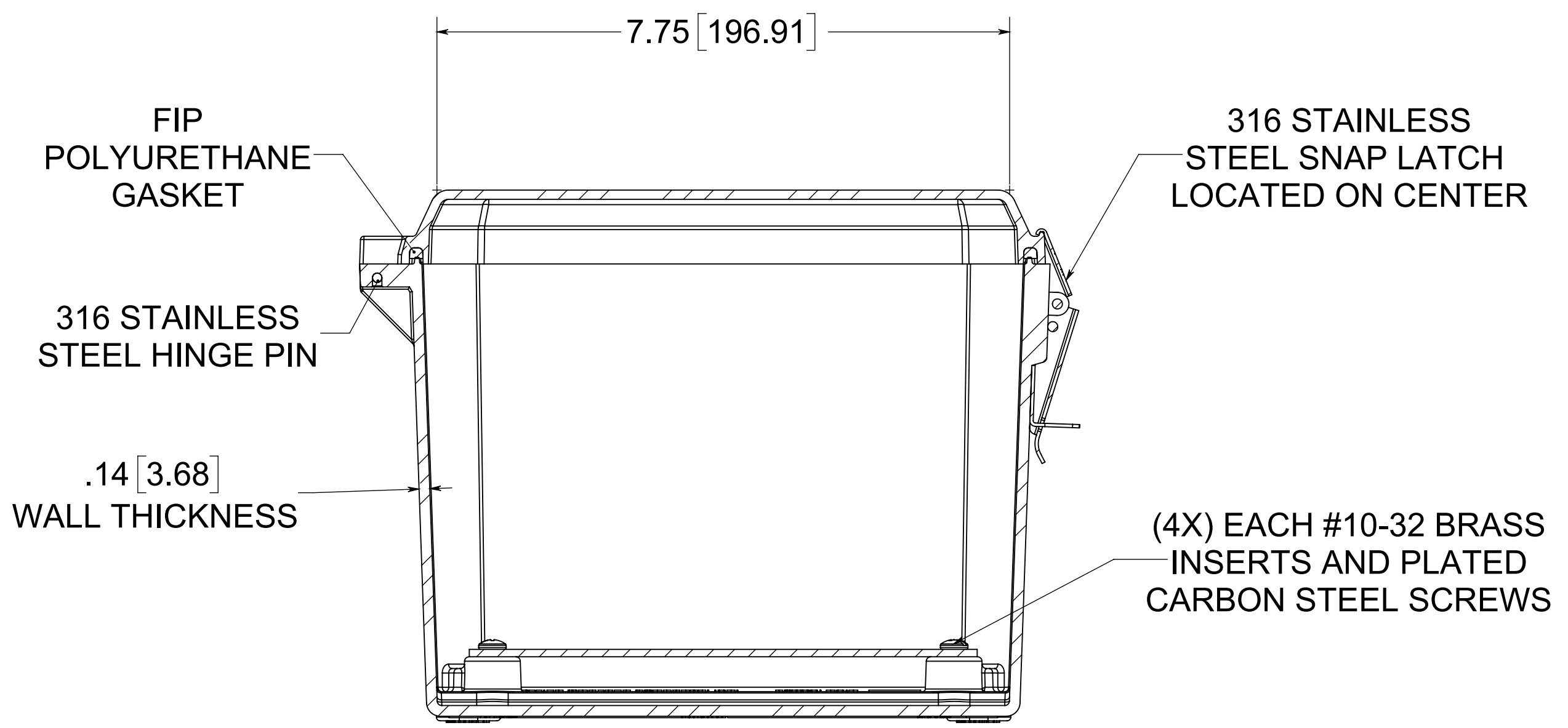
SECTION A-A
