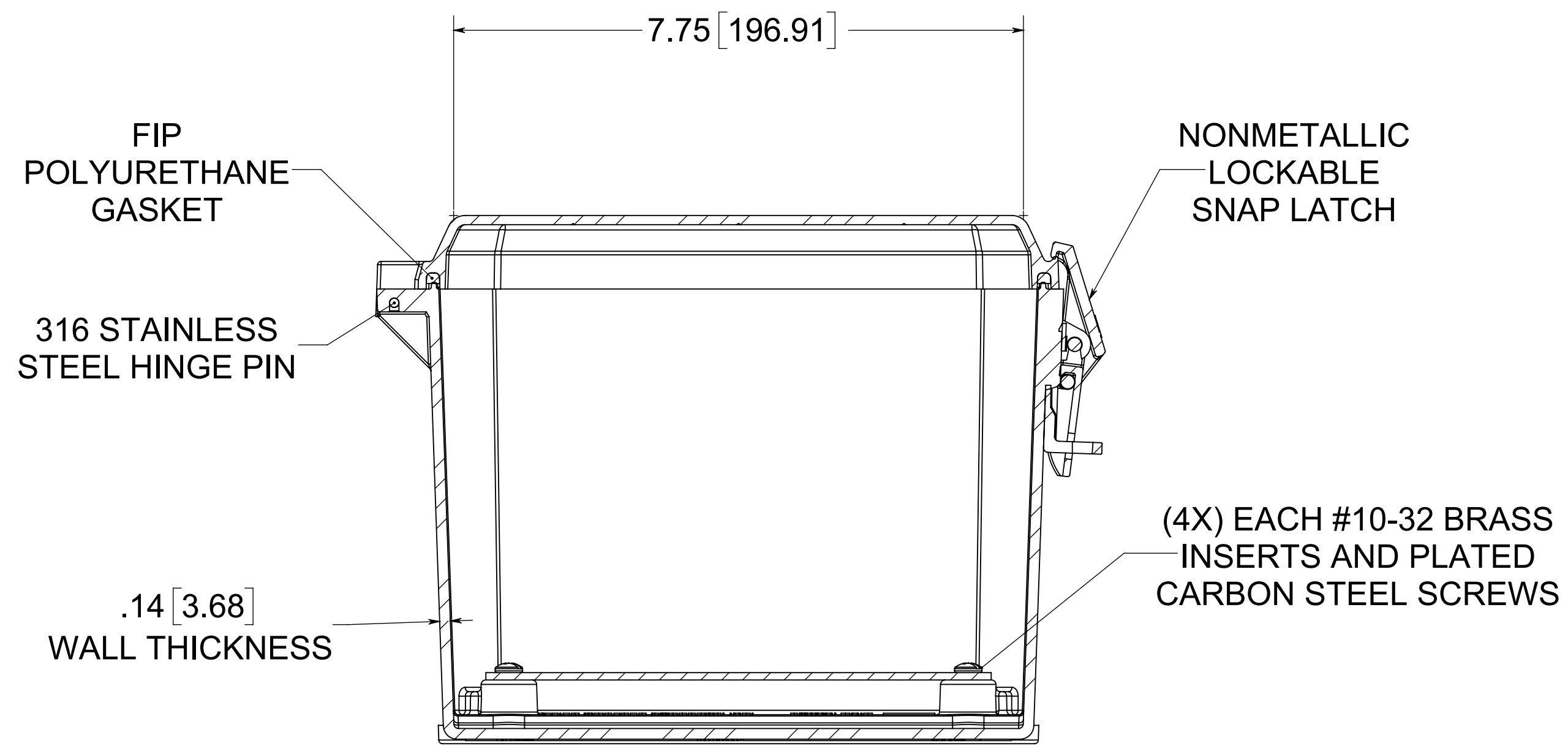
SECTION A-A
