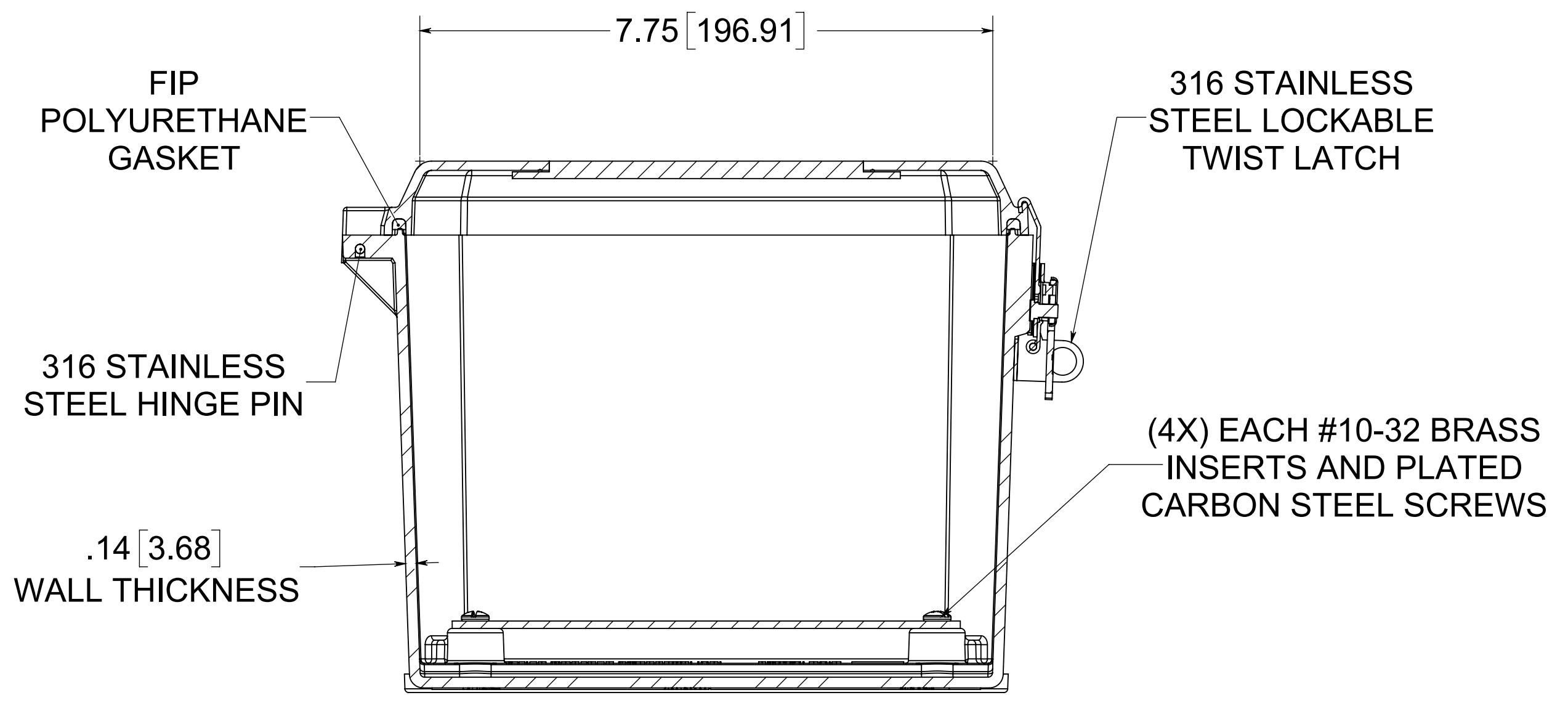
SECTION A-A
